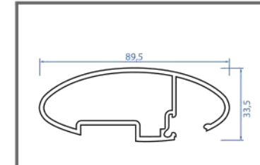
TK 901
