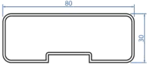
TK 800 80x30 Sabit Küpeşte Profili 80x30 Fixed Balustrade Profile
