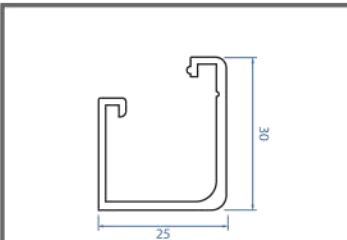
TK 3025
