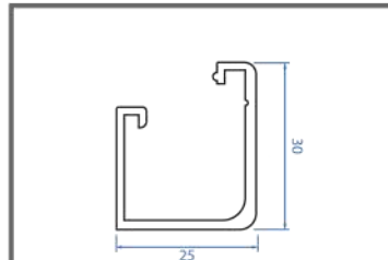
TK 3025
