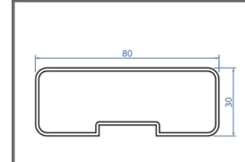
TK 800
