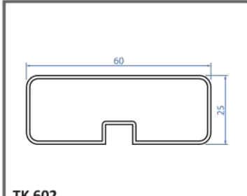
TK 602
